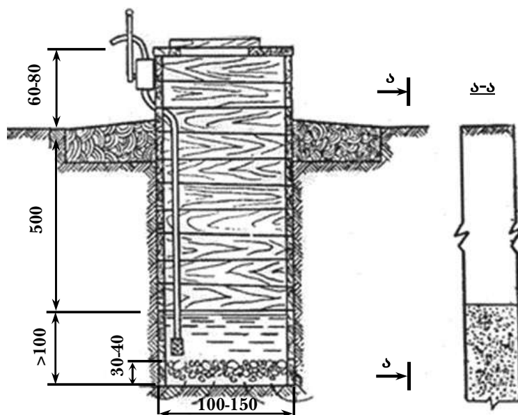
ნახ. 1. შახტური ჭა მისი კედლების ფიცრული ფარებით გამაგრების შემთხვევაში
