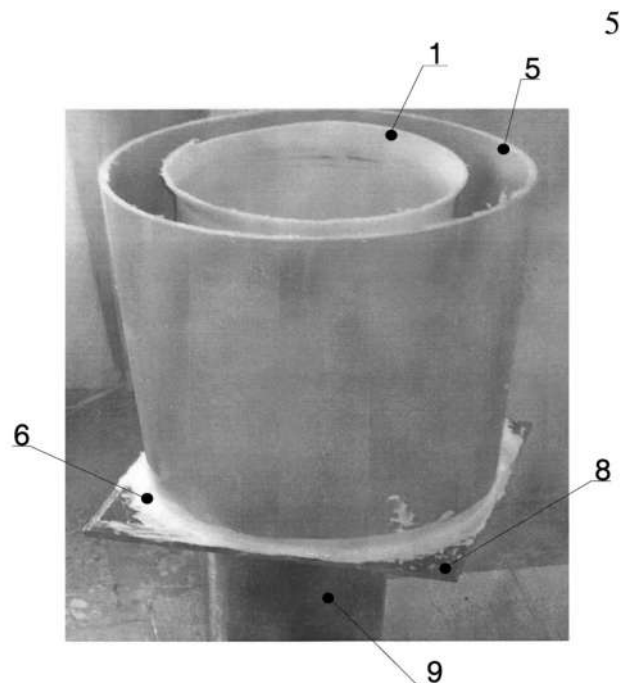
ნახ. 2. ფეთქებადი ნივთიერების ტესტირების სქემა (ა) და ტყვიის ცილინდრზე გამოსაცდელი მუხტის მასრის აწეობის ხედი (ბ): 1 - პლასტმასის მილი; 2 - გამოსაცდელი ფეთქებადი ნივთიერება; 3 - შუალედური დეტონატორი; 4 - ელექტროდეტონატორი; 5 - წყალშეუღწევი თხელი გარსი; 6 - პერმეტიკი; 7 - წყალი; 8 - ფოლადის ფირფიტა; 9 - ტყვიის ცილინდრი (კრეშერი); 10 - ფოლადის ფილა
