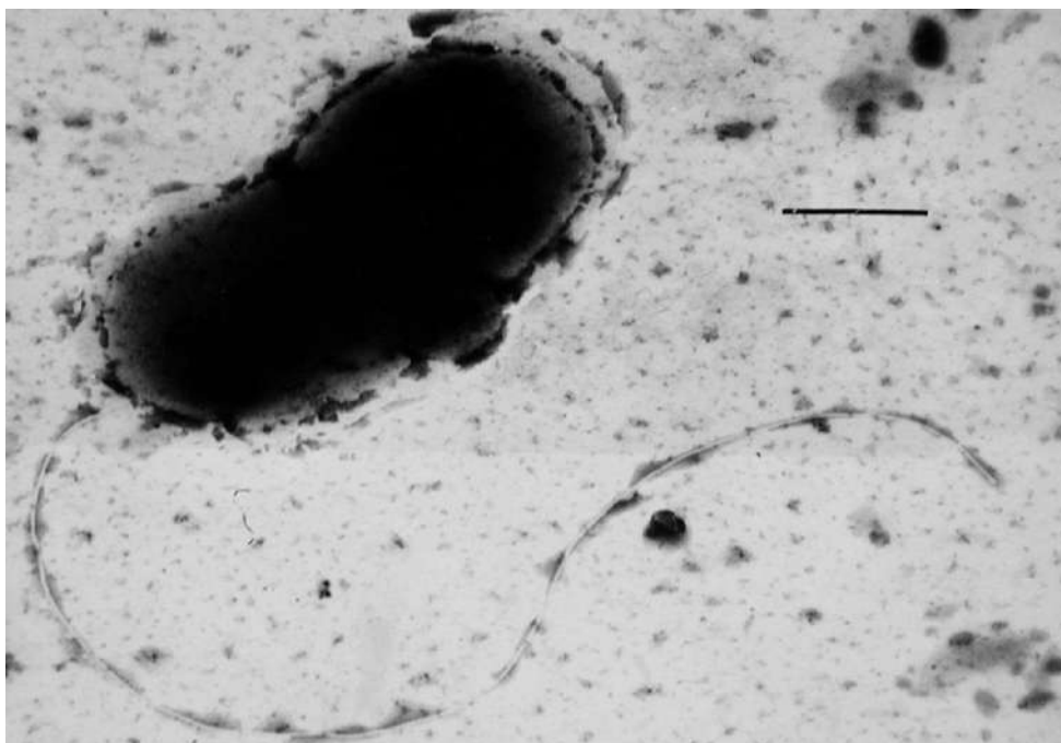
ნახ. 2. ანაერობული ბაქტერია დესულფოვობრიო, რომელიც ანაერობულ პირობებში საბურღი ხსნარში \text{H}_2\text{S} წარმოქმნის
