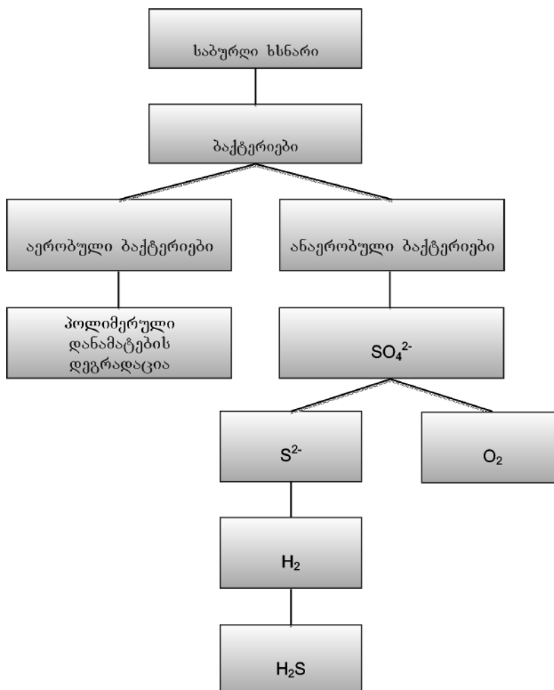
ნახ. 1. სამუშაო სხნარზე ბაქტერიების ზემოქმედების სქემა
