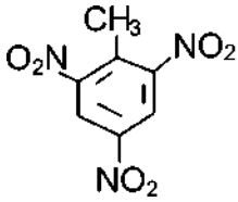
2, 4, 6 – ტრინიტროტოლუოლი ტროტილი ამ შემთხვევაში მოლეკულათა სტრუქტურული
